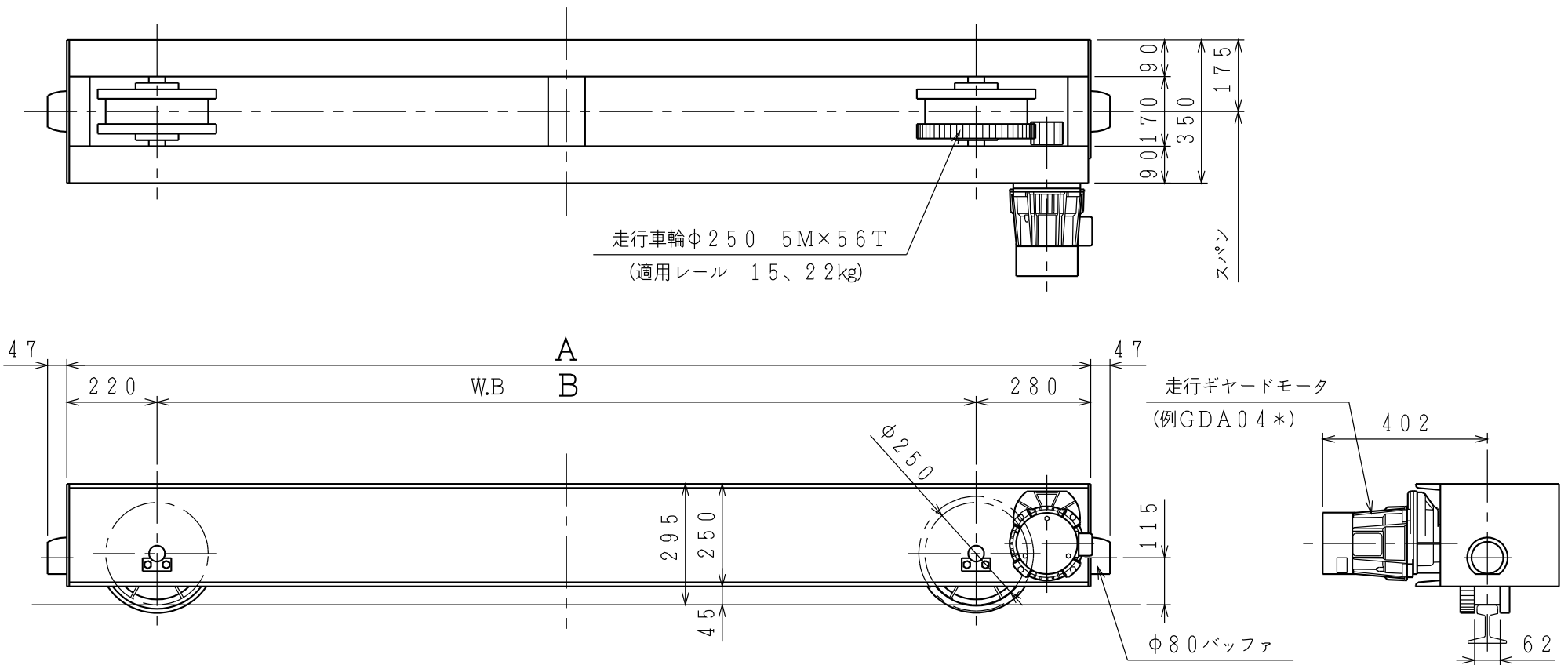
寸法 (mm)
