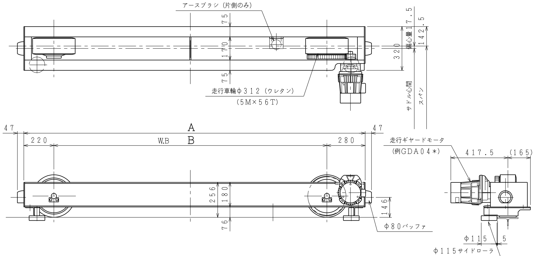
寸法 (mm)
