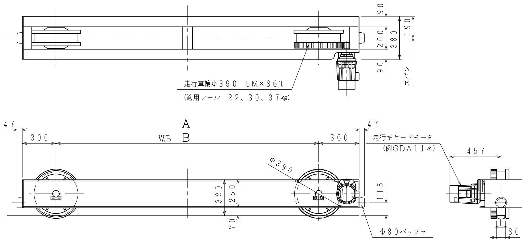
寸法 (mm)
