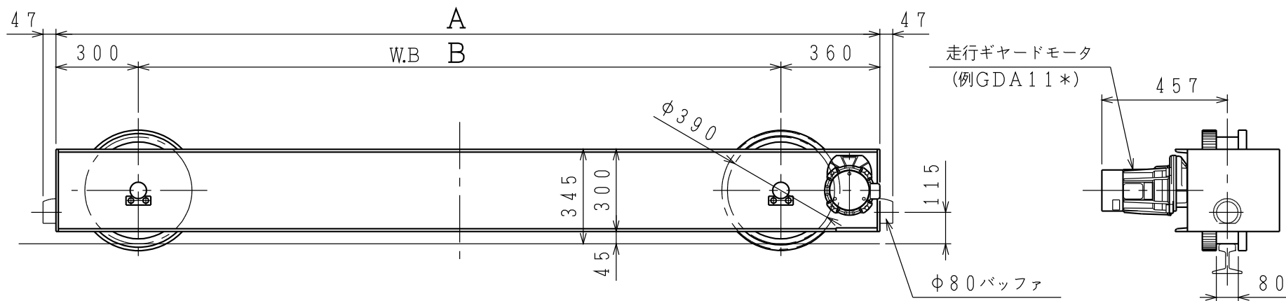
寸法 (mm)
