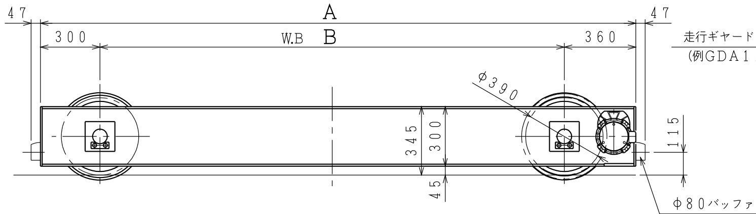
寸法 (mm)
