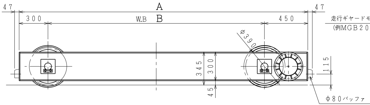
寸法 (mm)
