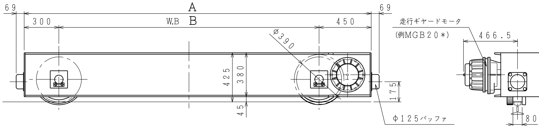
寸法 (mm)
