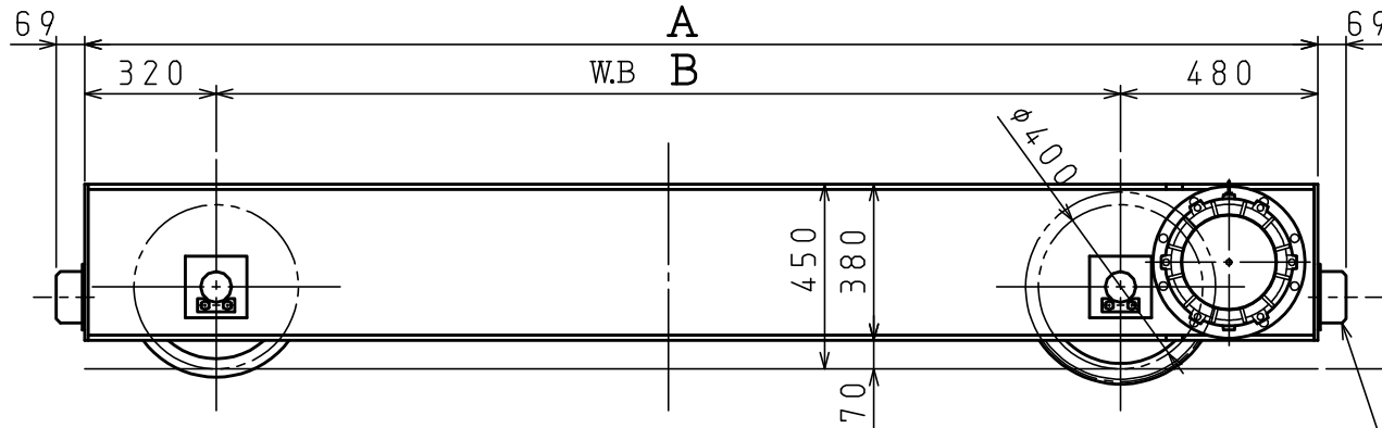
寸法 (mm)
