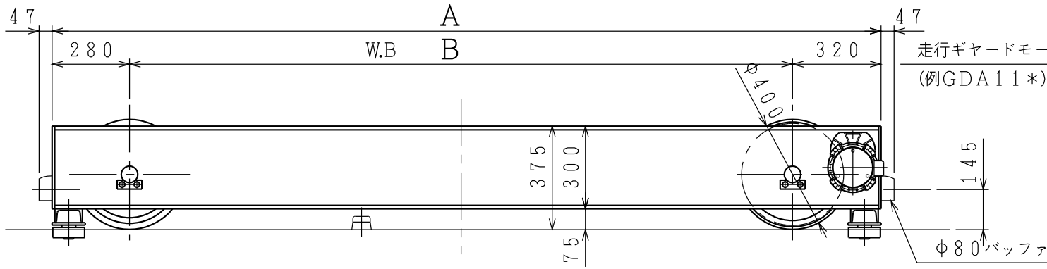
寸法 (mm)
